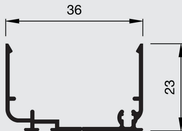
Seitenprofil mit Gewichtskasten vertikal
