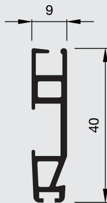
Untere Führungsschiene
