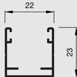
Obere Führungsschiene
